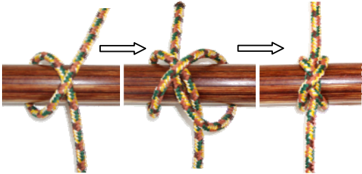
Констриктор
