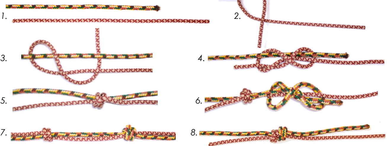
Стивидорный узел
