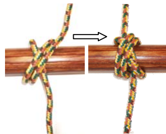
Двойной Констриктор
